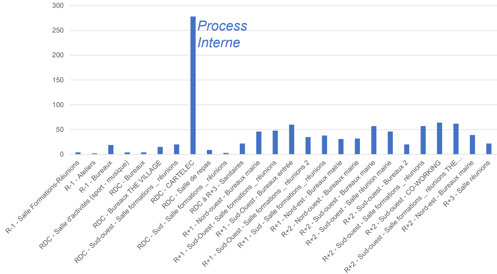
Nombre d'heures > 28°C en période d'occupation
