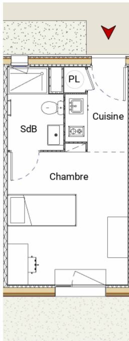
1 Plan type T1 1 : 100
