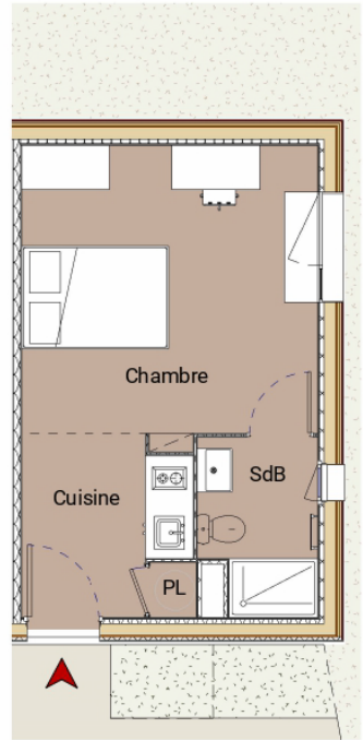
2 Plan type T1 bis 1 : 100
