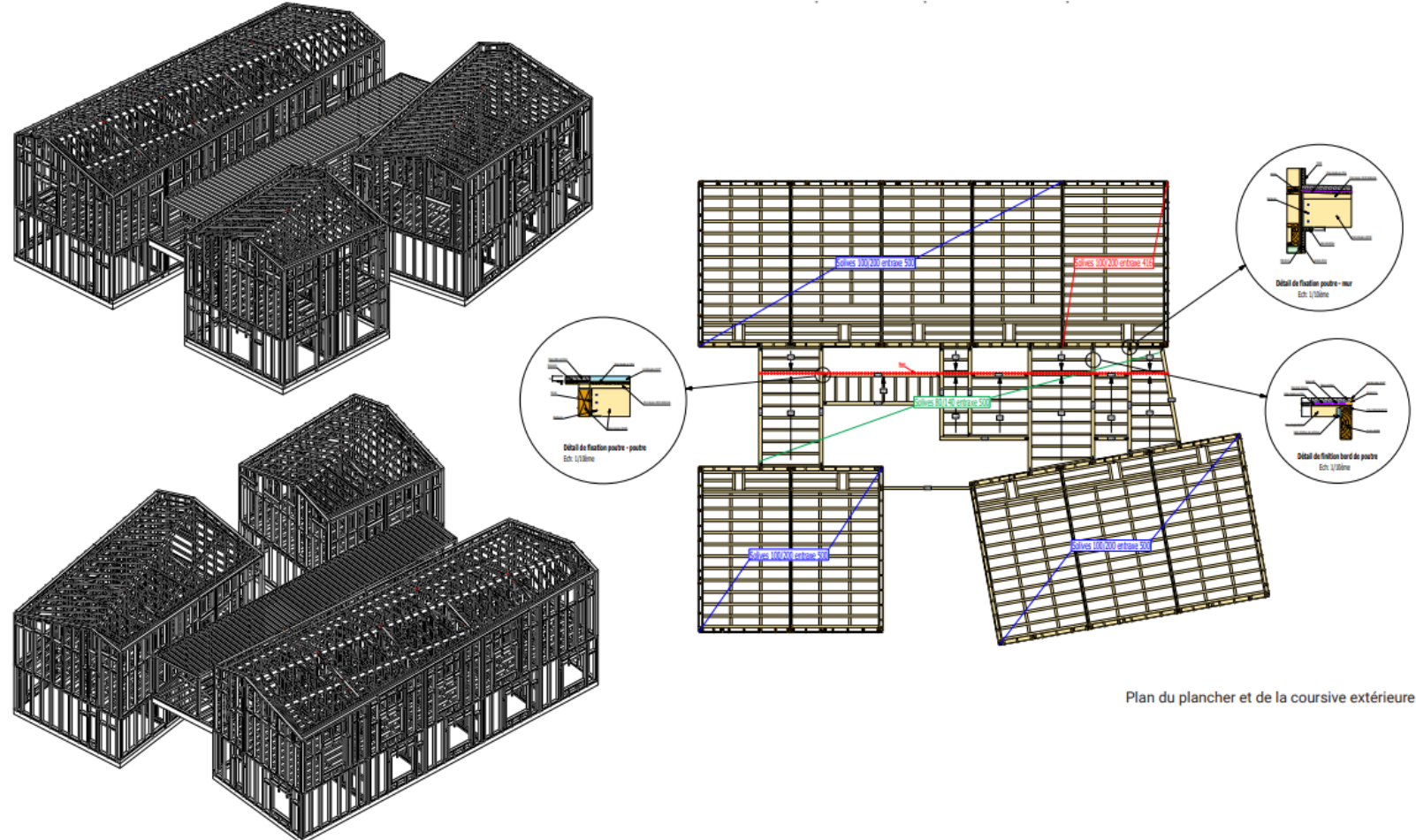
Vues axonométriques de la structure bois
