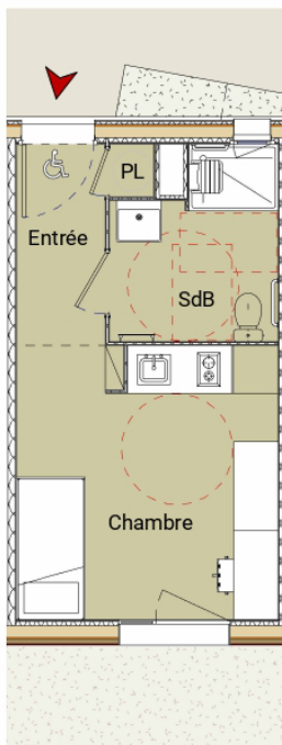
3 Plan type T1 PMR 1 : 100
