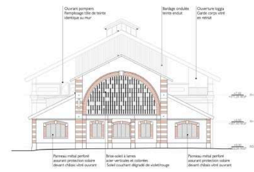
Façade ouest
