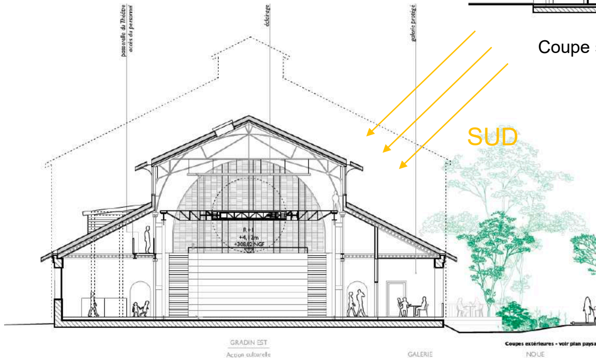
Coupe nef et bas côtés
