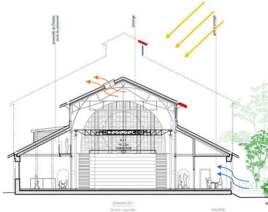
Ombres portées – 15/05 à 10h
