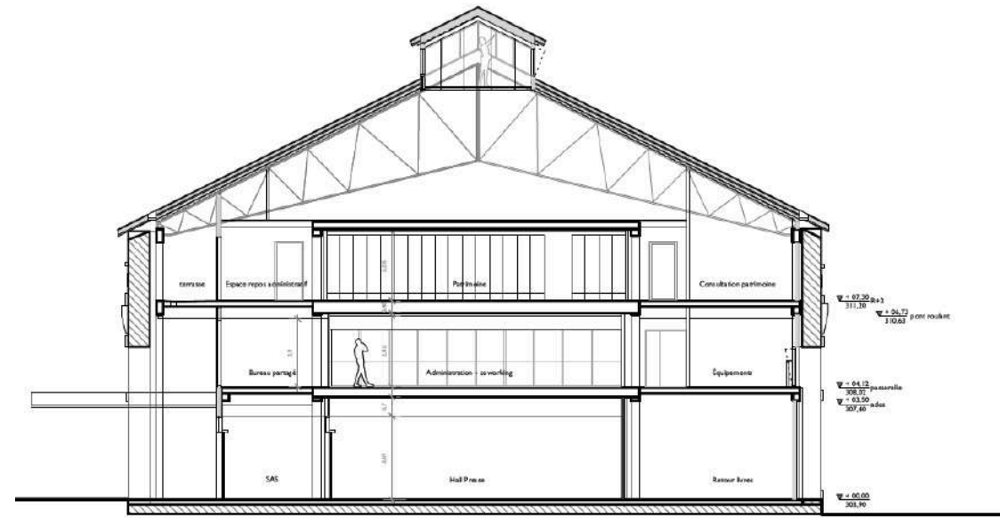
Coupe sur pavillon central
