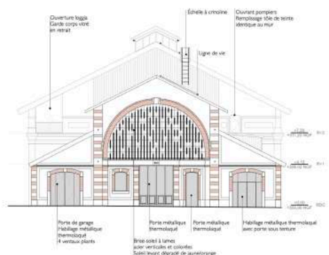
Façade est
